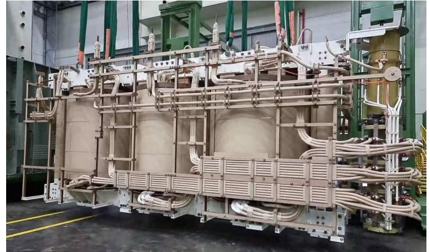
AUTO, 450 MVA- 400/138/33 kv. COREA DEL SUR
